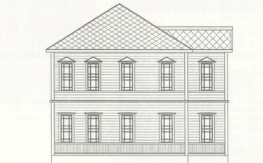
東側立面図
